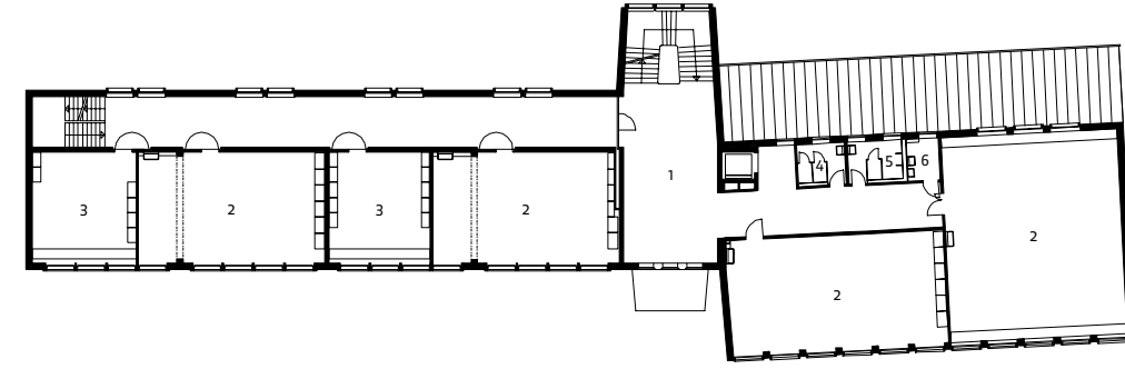
Erstes Obergeschoss
