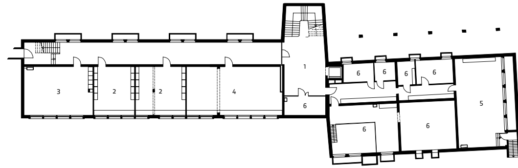
Untergeschoss
