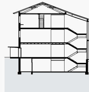
Querschnitt
