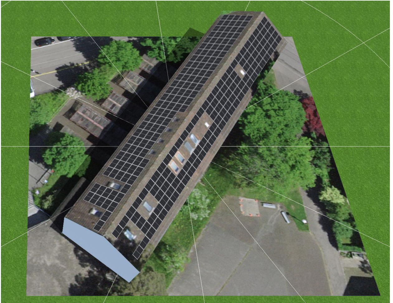
Planung der Belegung für das Schulhaus Büelwiesen
