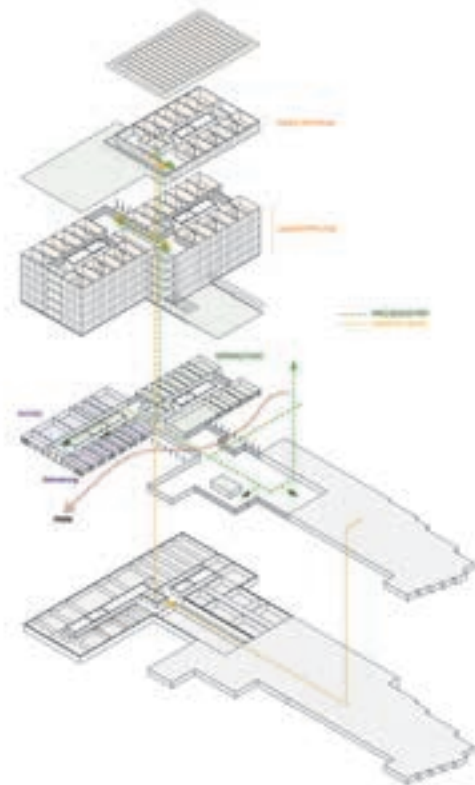
Schema Wege
