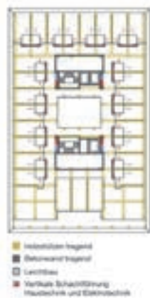
Schema Statik und Haustechnik
