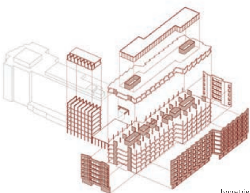
Isometrie
