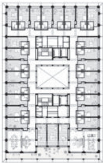
Regelgeschoss, 2.-5. Obergeschoss
