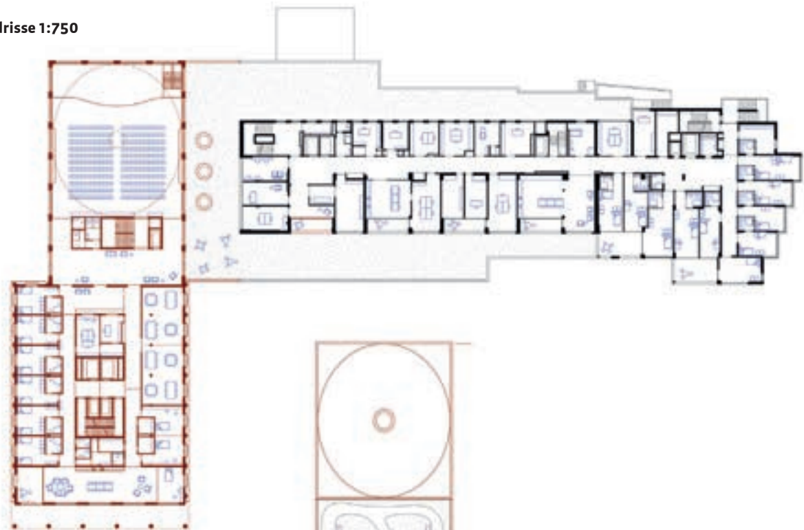
1. Obergeschoss
