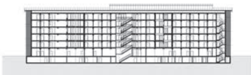
Längsschnitt
