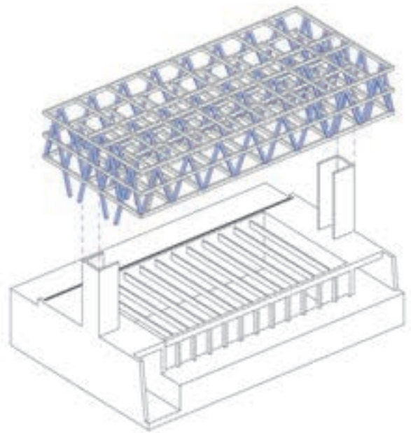
Tragwerk mit Holzraumfachwerk
