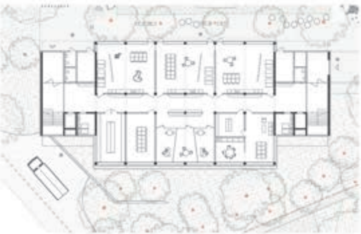
Erdgeschoss
