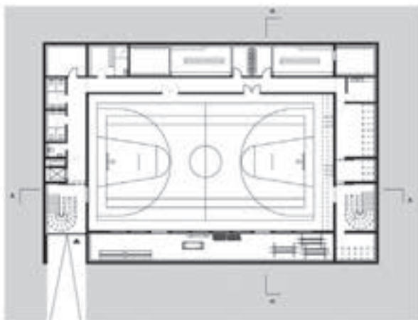
2. Untergeschoss
