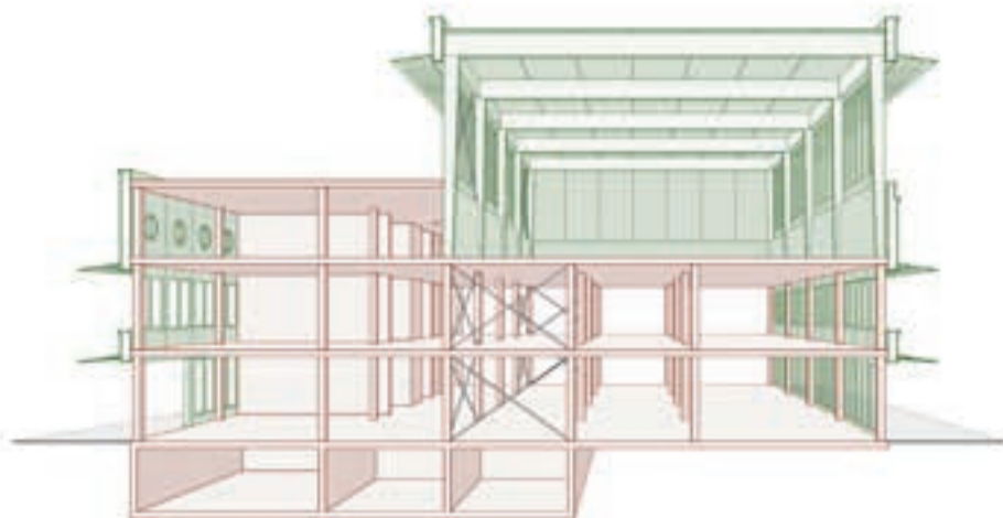
Schnittperspektive
