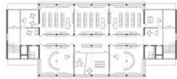
1. Obergeschoss
