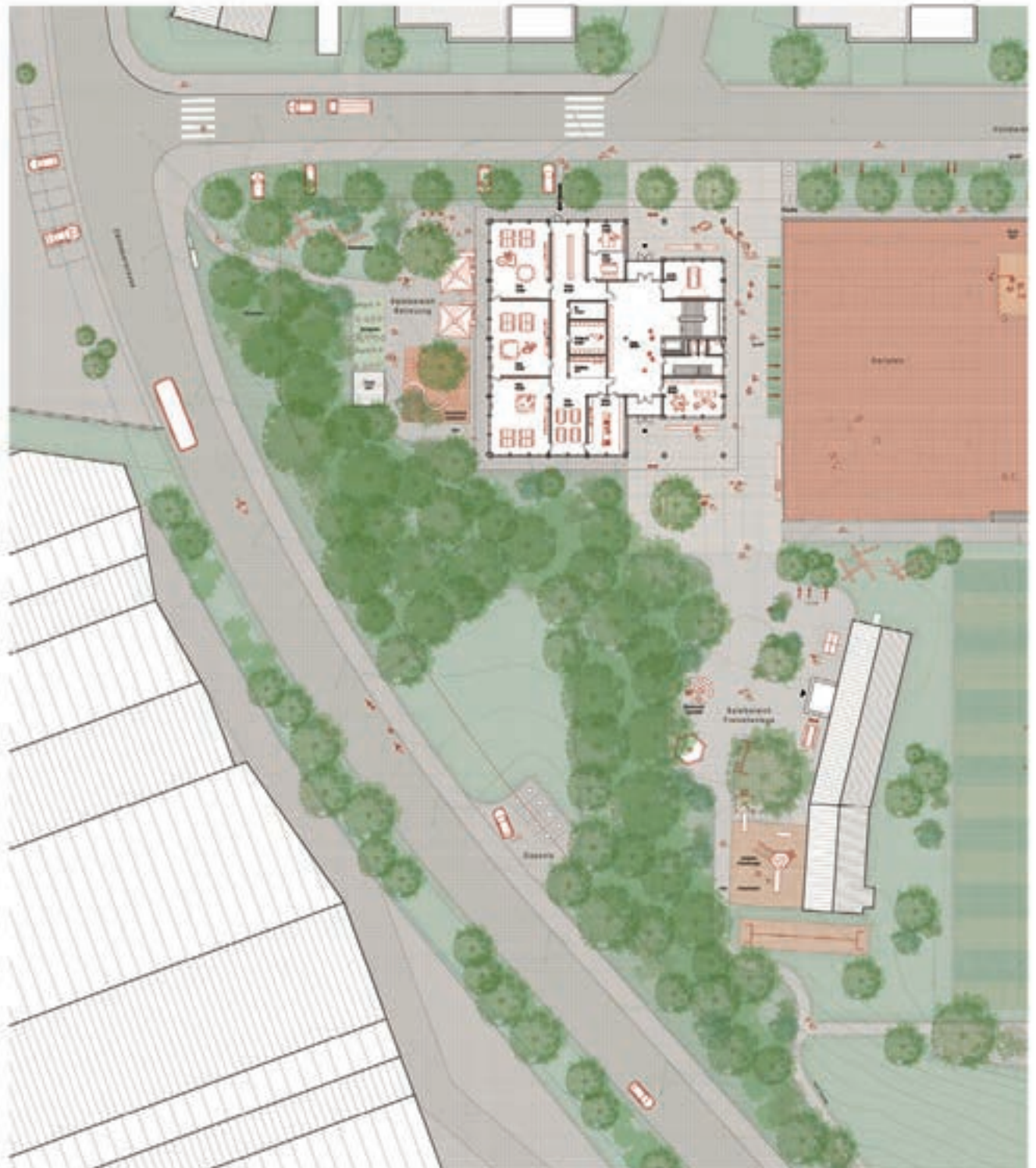
Erdgeschoss mit Umgebung
