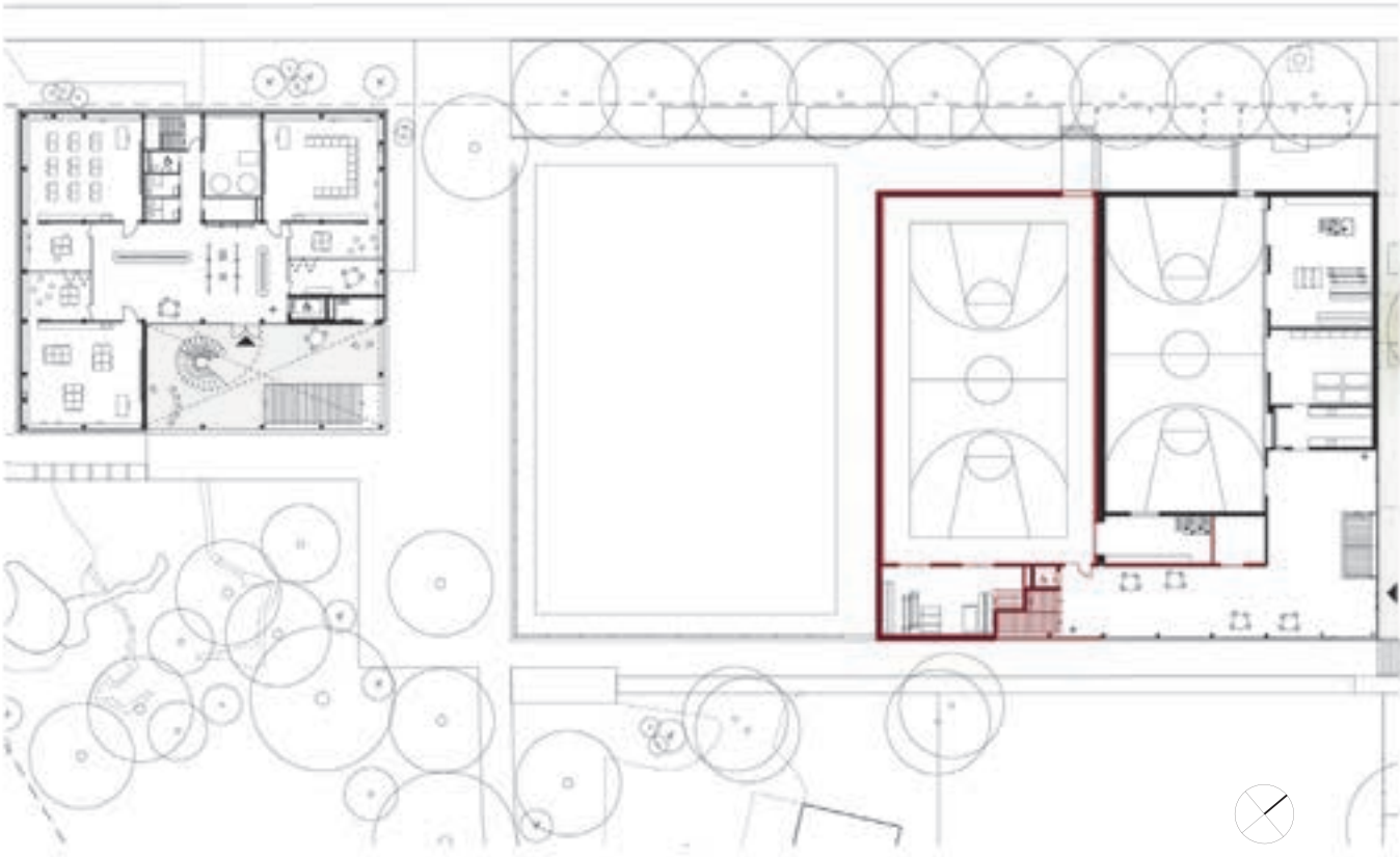
1. Obergeschoss
