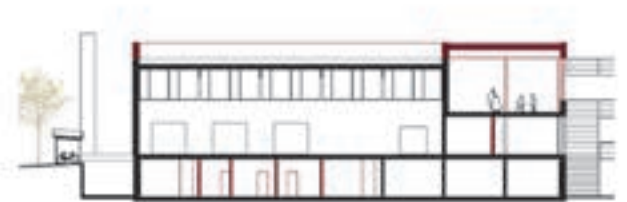
Schnitt Mehrzweckhalle
