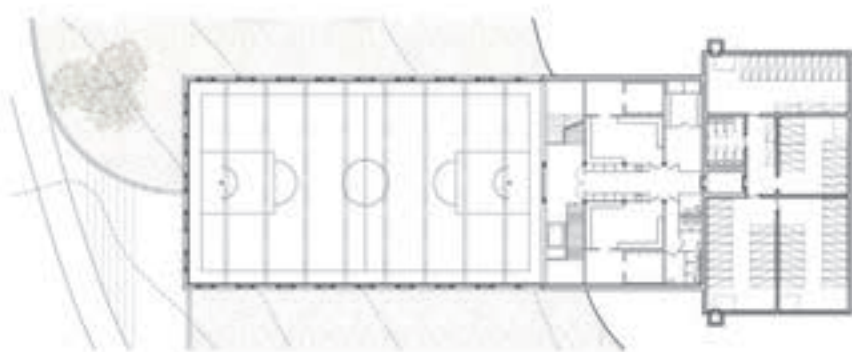
Garderobengeschoss
