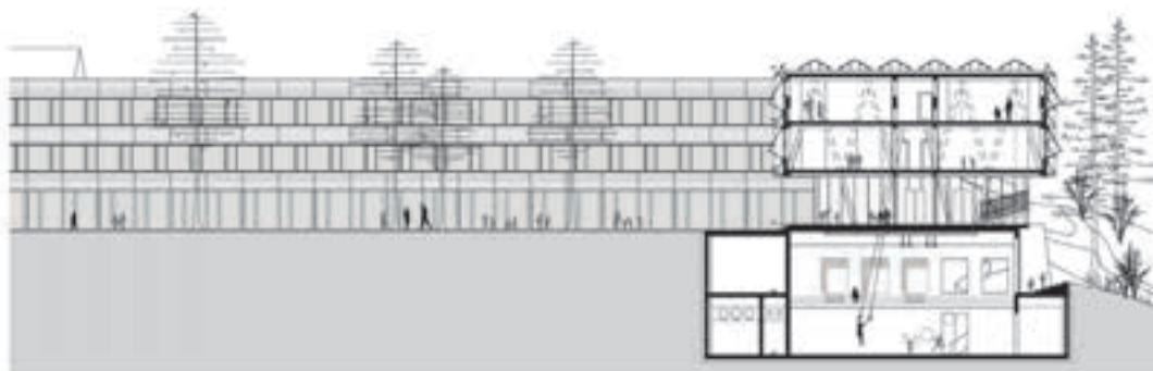
Querschnitt
