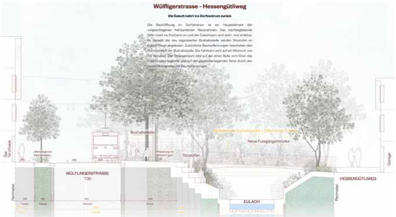
Schnitt durch die Eulach, Wülfingerstrasse und Hessengütlweg
