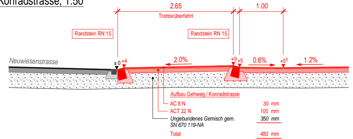
Schnitt Konradstrasse, 1:50
