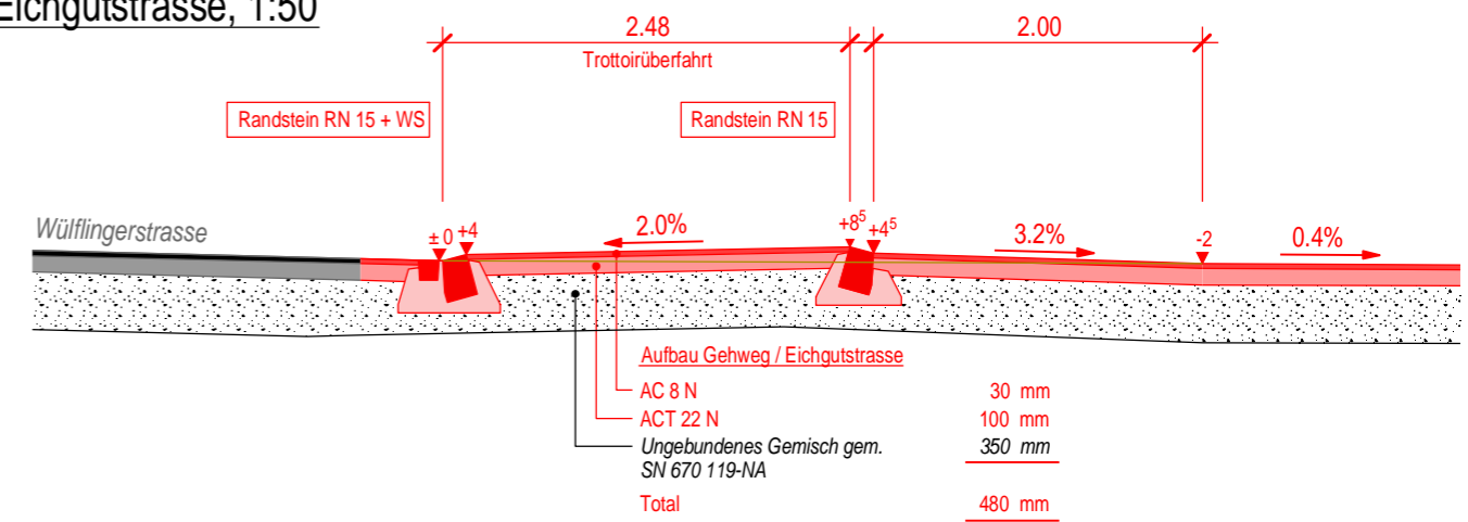
Schnitt Eichgutstrasse, 1:50
