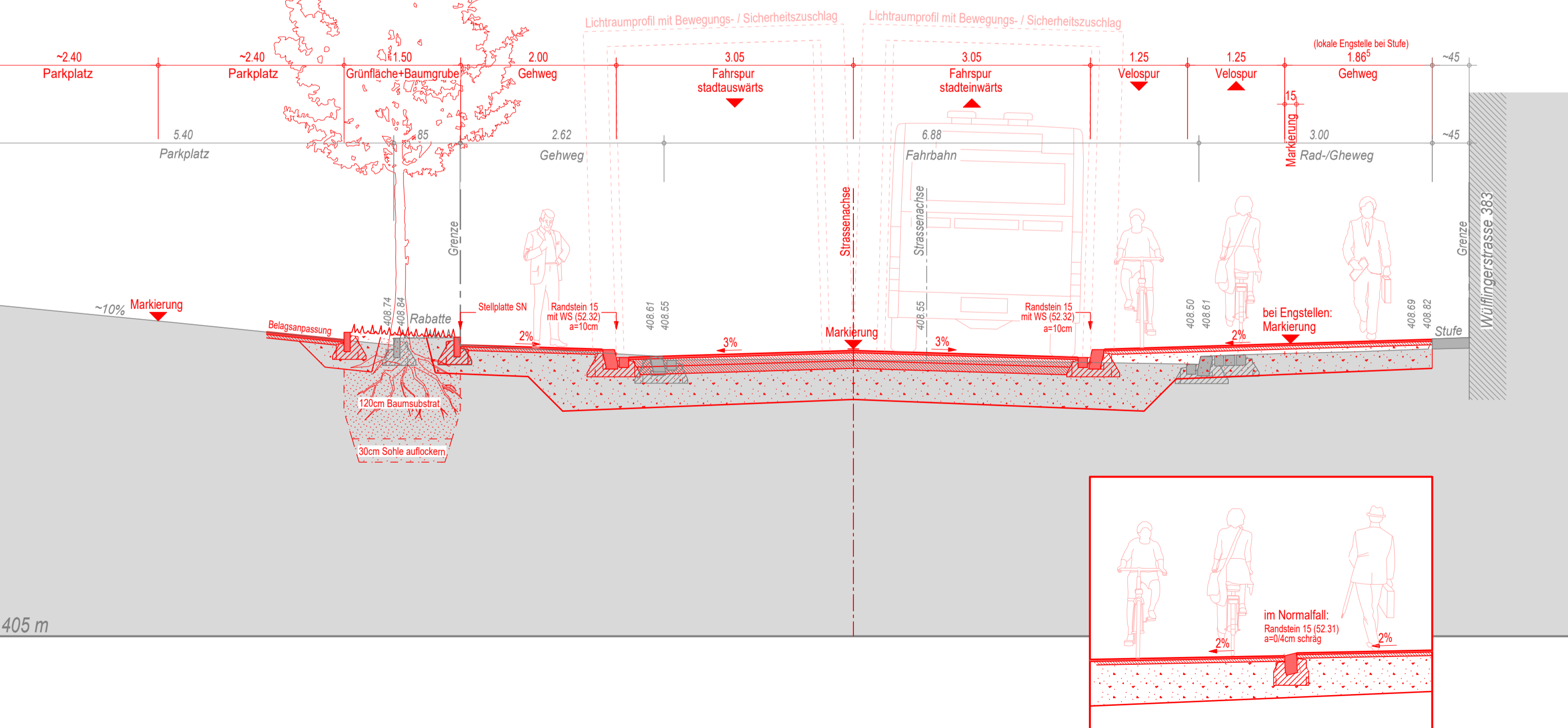
Normalprofil B-B, 1:50
